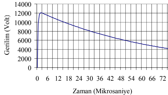
Şekil 4: Darbe üreticinin çıkış dalga şekli.
