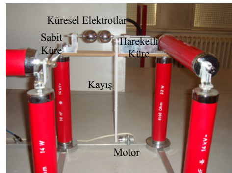
Şekil 5: Darbe üreticinin küresel elektrot sistemi
