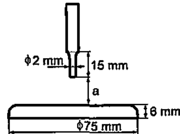
Şekil 1. Hesaplarda göz önüne alınan çubuk-düzlem elektrot sistemi
