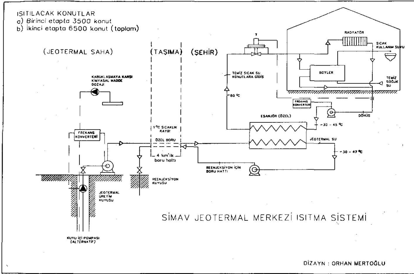
ŞEKİL-10: Simav jeotermal merkezi ısıtma sistemi
