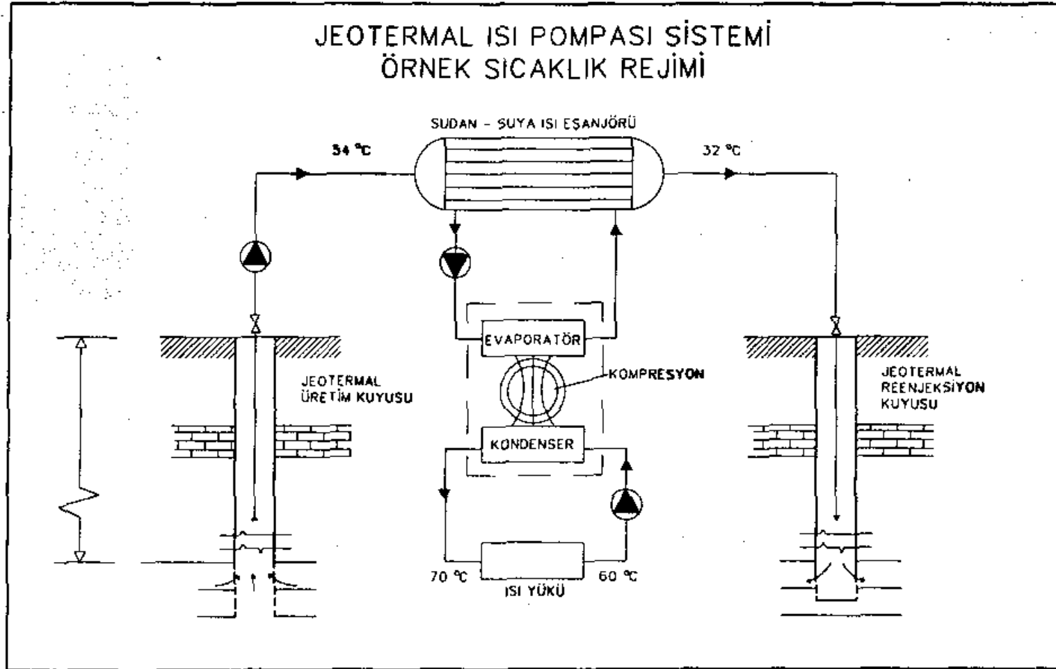
ŞEKİL-7: Jeotermal ısı pompası sistemi örnek sıcaklık rejimi
