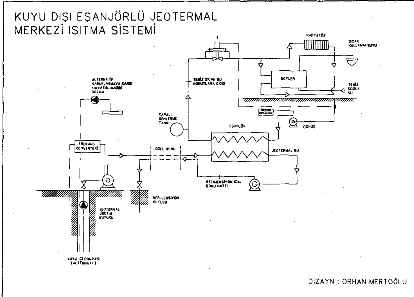
ŞEKİL-6: Kuyu dışı eşanjörlü jeotermal merkezi ısıtma sistemi
