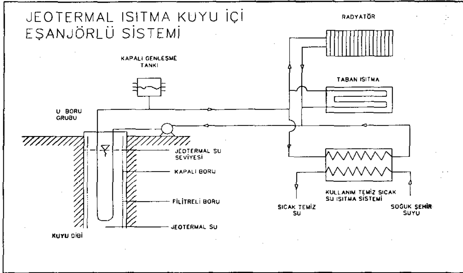
ŞEKİL-5: Kuyu içi eşanjörlü jeotermal ısıtma sistemi
