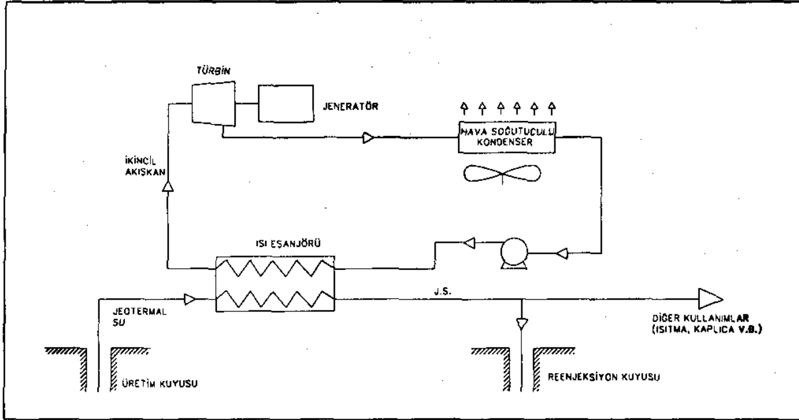
ŞEKİL-4: Binary çevrim jeotermal elektrik üretim sistemi
