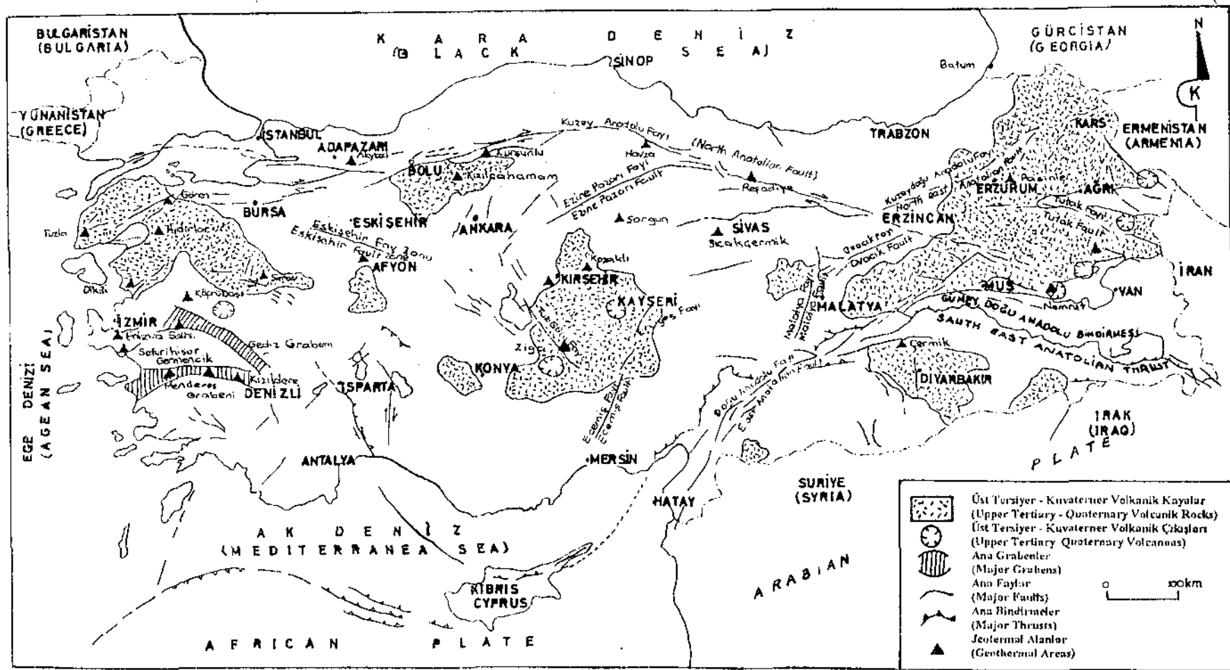
ŞEKİL-8: Türkiye'nin neotektoniği- volkanik etkinliği ve jeotermal alanları
