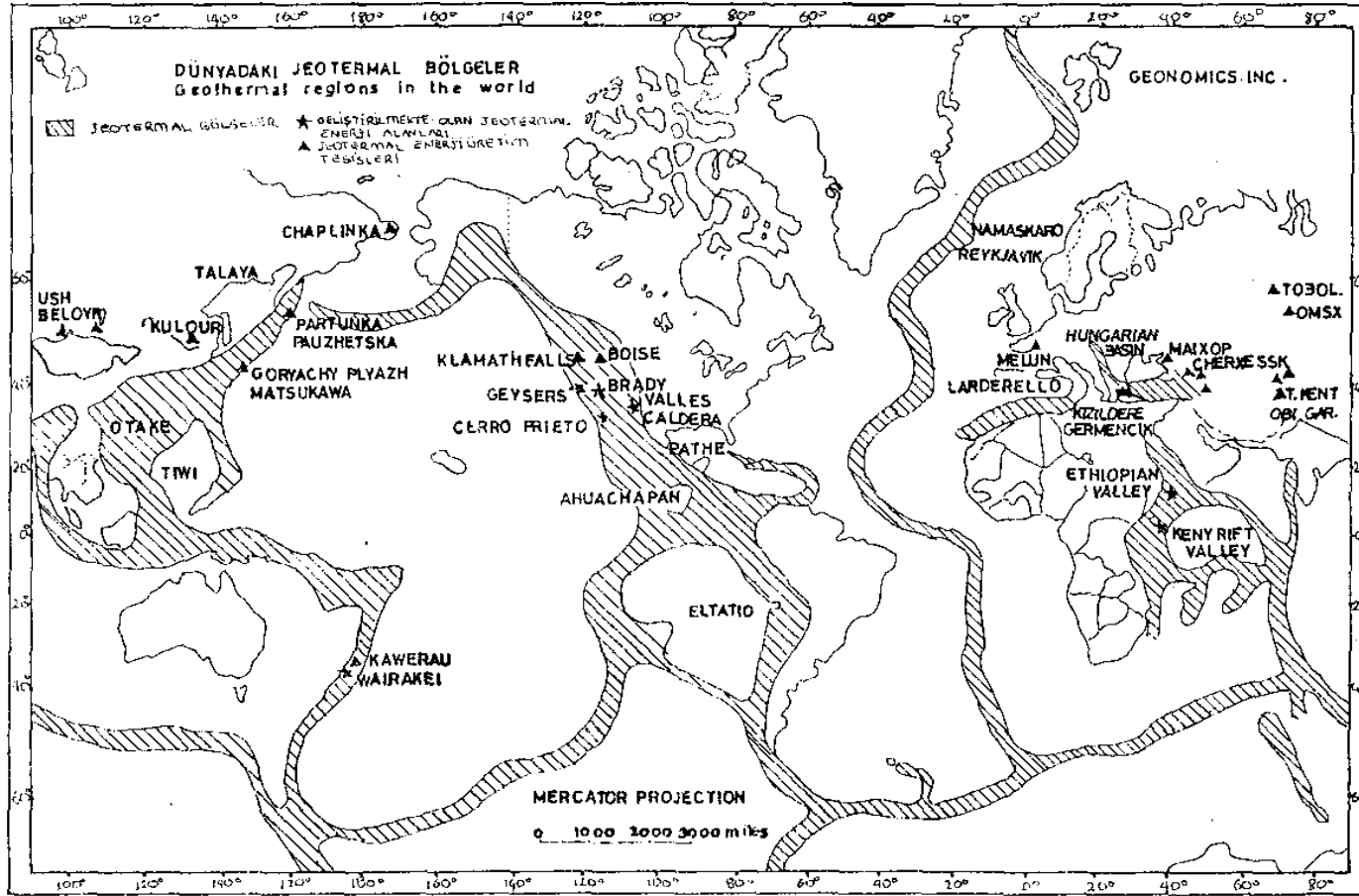
ŞEKİL-1: Dünyadaki jeotermal kuşaklar
