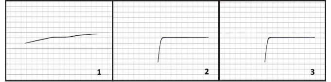
Şekil 4.12. Orijinal-2 LF353 1,2 ve 3 pinleri VI eğrileri.
