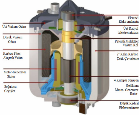
Şekil 3. Volan enerji depolama ünitesinin kesit şeması[13]
