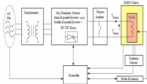
Şekil 2. Tipik bir SMES sistemi bileşenleri[12]
