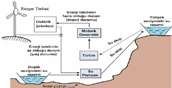
Şekil 4. Pompalı hidroelektrik enerji depolama akış diyagramı
