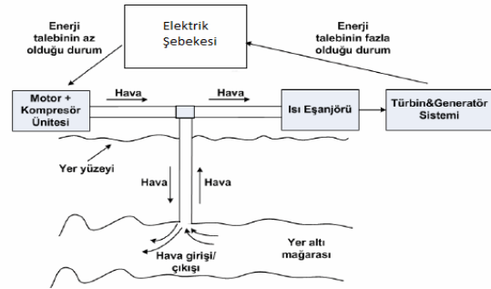
Şekil 5. Sıkıştırılmış hava enerji depolama akış diyagramı[17]
