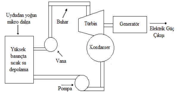
Şekil 6. Isıl enerji depolama blok diyagramı[20]
