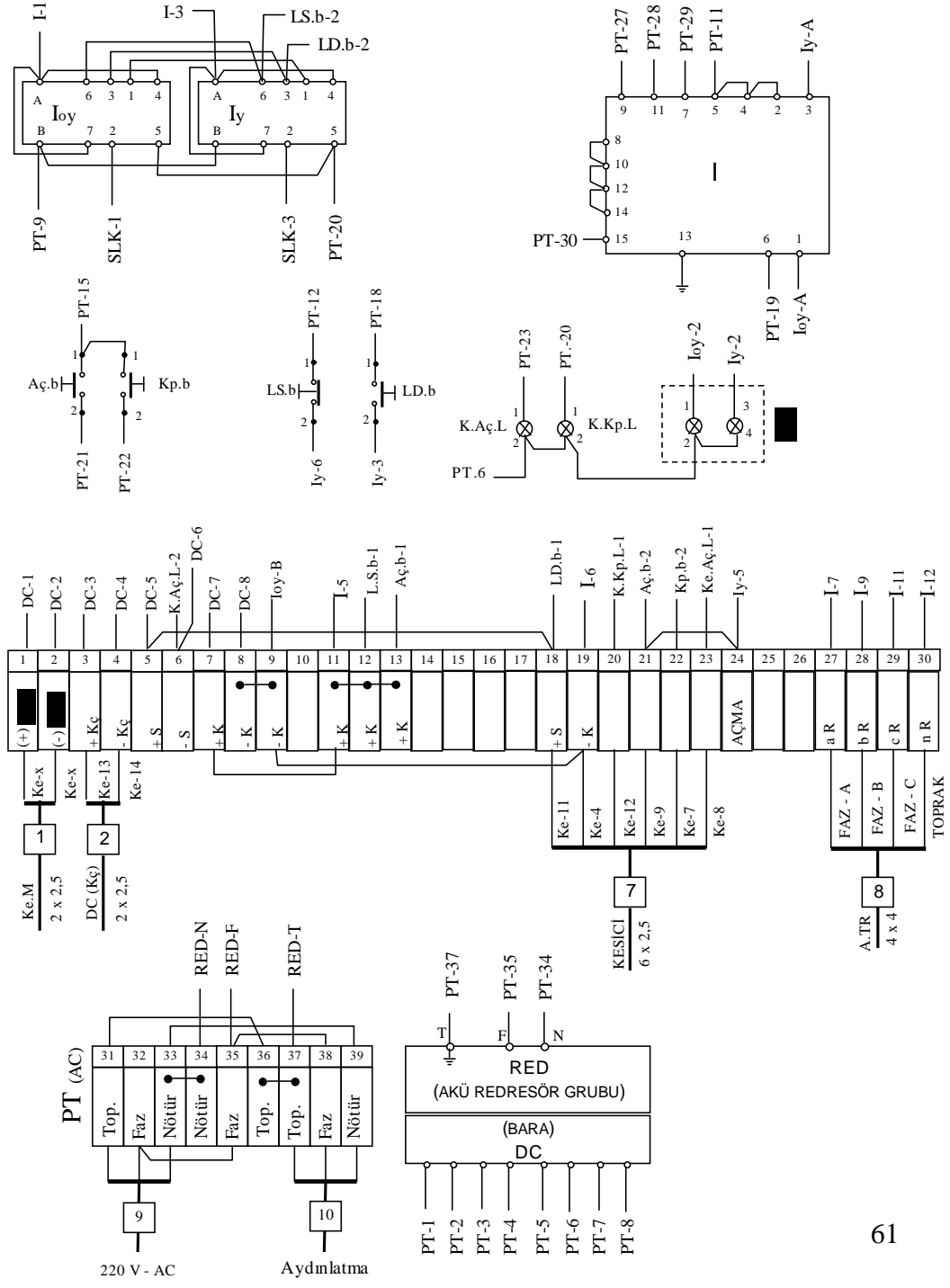
TİP:4 2 AA + Top ve Trafo Zati Koruma BAĞLAMA ŞEMASI
