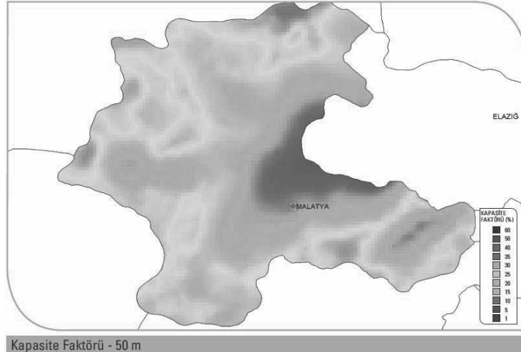
Harita 10- Malatya İli Rüzgâr Enerjisi Kapasite Faktörü Dağılımı 50 m
