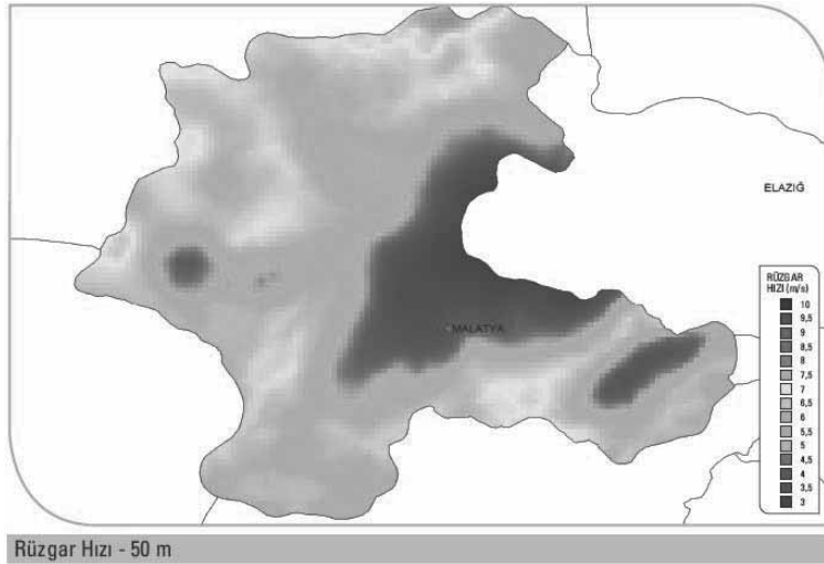
Harita 9 - Malatya İli Rüzgar Hızı Dağılımı 50 Metre
