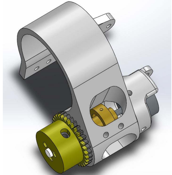
Şekil 4: Potansiyometre bağlantı montajı.
