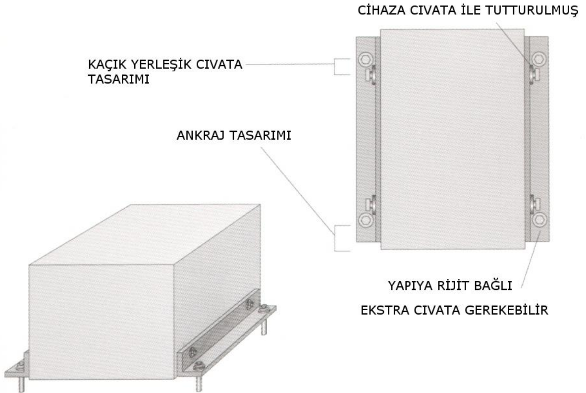
Şekil-3 Donanımın ileve takviye ile dösemeye sabitlenmesi*
