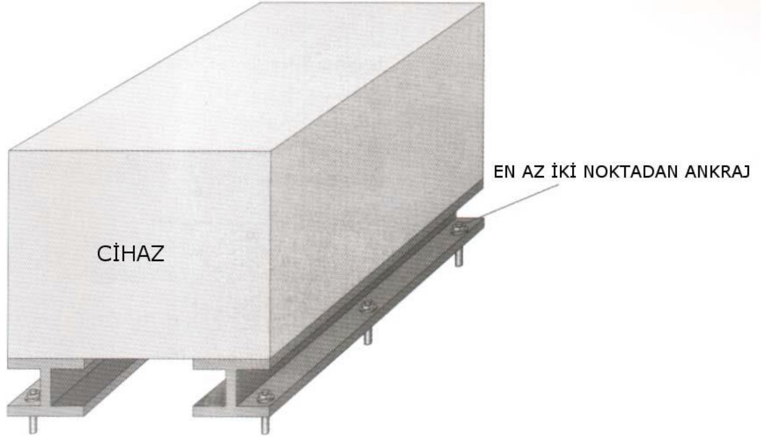
Şekil-2 Donanımın altına yapılan ilave şasiden döşemyte sabitlenmesi*
