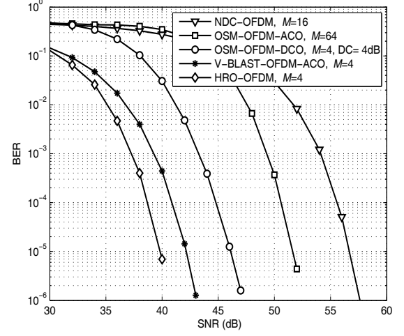
Şekil 3: Kurulum A İçin Tablo 2'deki Sistemlerin BER Başarımları (2bit/s/Hz)
