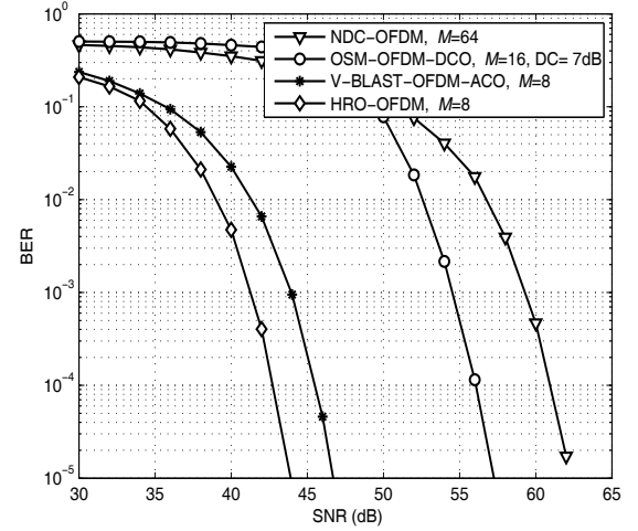
Şekil 4: Kurulum A İçin Tablo 2'deki Sistemlerin BER Başarımları (3bit/s/Hz)
