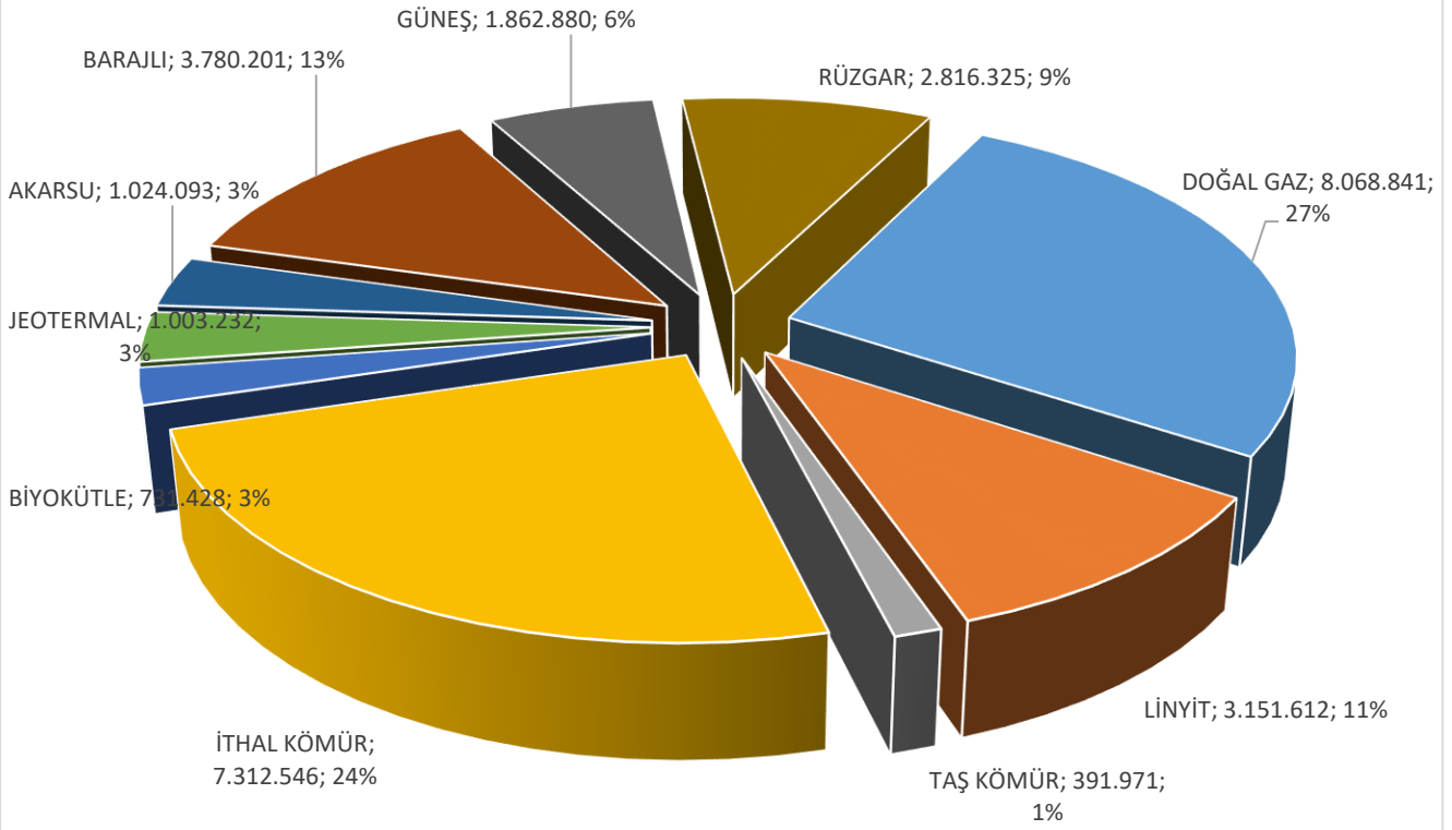
Ocak 2025 Aylık Üretimin Kaynaklara Göre Dağılımı (MWh)
