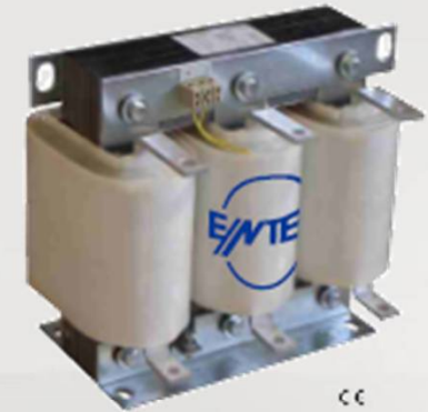
Harmonik Filtre Reaktörü
