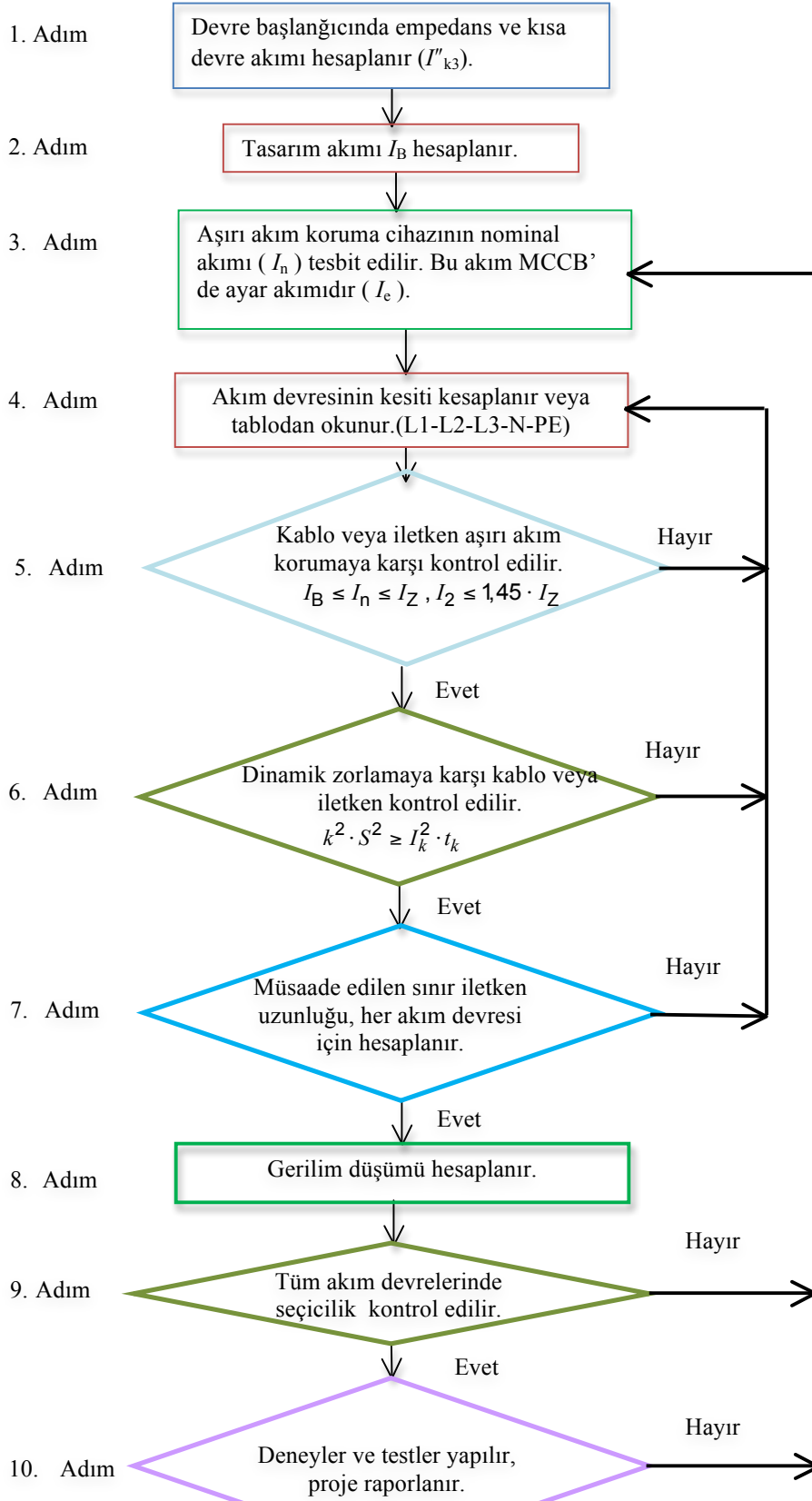
Şekil 2 – Akım devresi koordinasyonu ve işletme cihazlarının belirlenmesi
