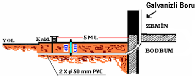
Örnek 3: Telekom Şebekesi İrtibatı.
