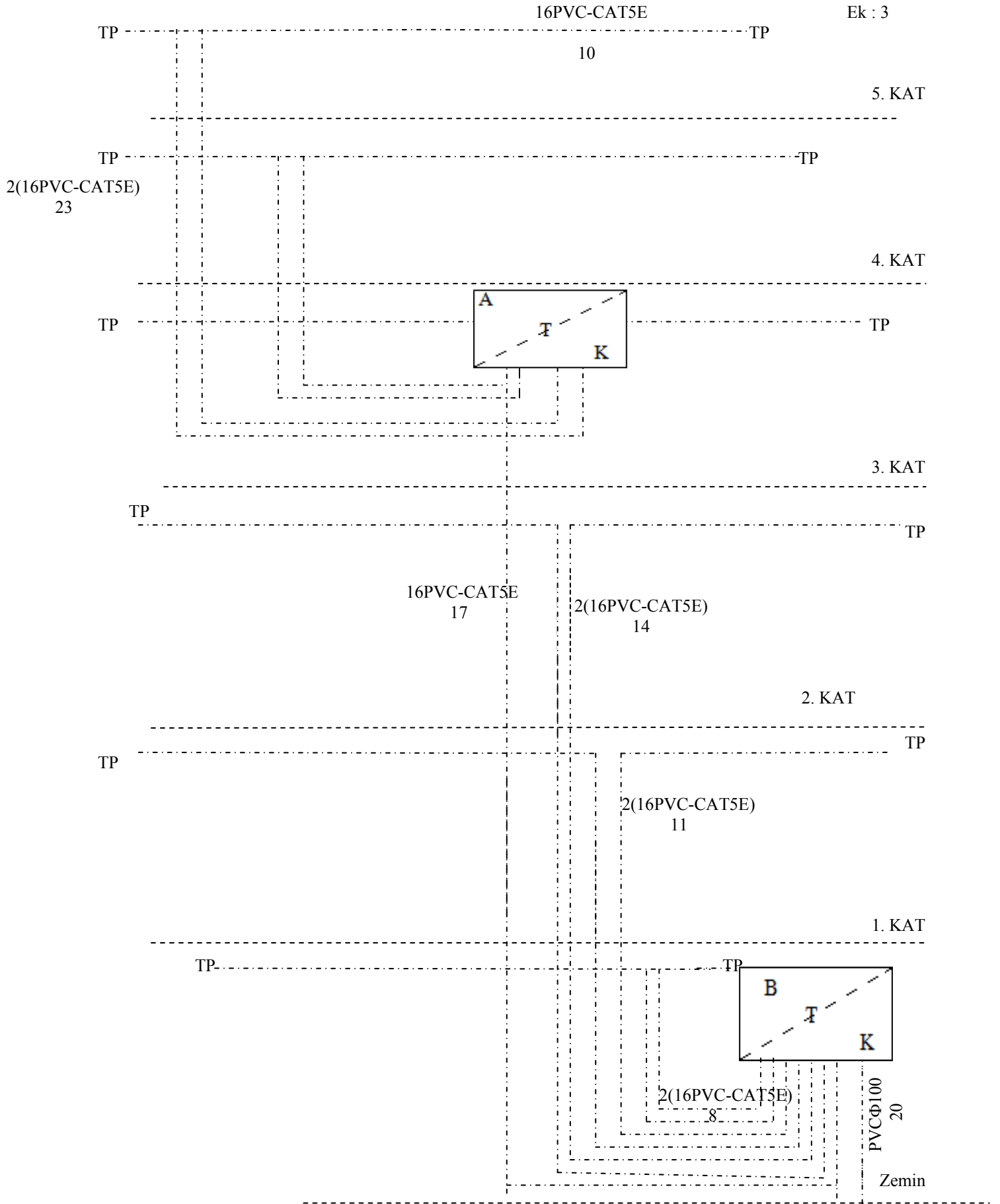
KOLON DAĞITIM ŞEMASI
