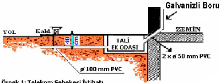
Örnek 1: Telekom Şebekesi İrtibatı.
