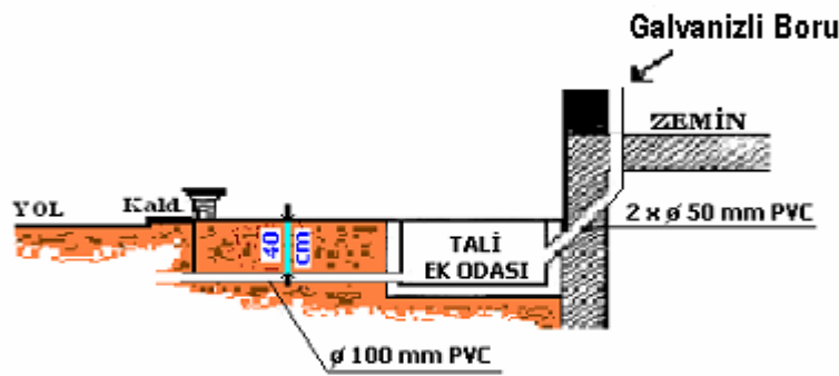
Örnek 2: Telekom Şebekesi İrtibatı.
