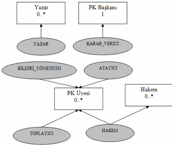
Şekil 5: Etmen modeli
