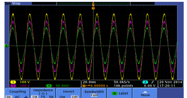
Şekil 11: %22'lik Gerilim Çökmesi Tam Yük Grafikleri (Sarı: Çıkış Gerilimi, Mor: Giriş Gerilimi, Yeşil: Giriş Akımı)
