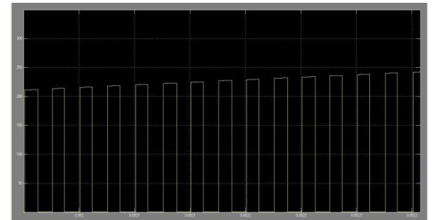
Şekil 25: Gerilim Kabarması Durumu, Yarı Yük, Pozitif Çevrim DGM Anahtarlama-Benzetim
