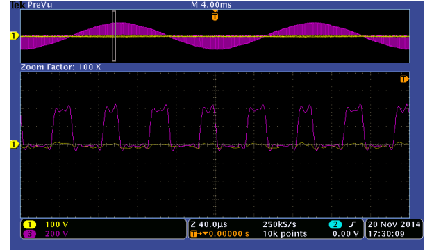
Şekil 24: Gerilim Kabarması Durumu, Yarı Yük, Pozitif Çevrim DGM Anahtarlama
