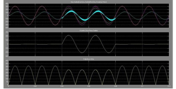
Şekil 10: %20'lik Gerilim Çökmesinin Gerilim-Akım Sinyalleri (Güç Katsayısı 0.8 Endüktif)
