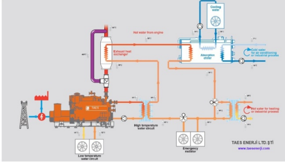
Şekil 5: Bir Trijenerasyon tesisi ana üniteleri
