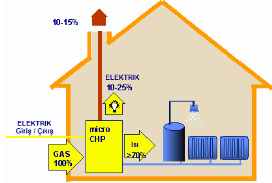
Şekil 3: Mikrokojenerasyon uygulaması
