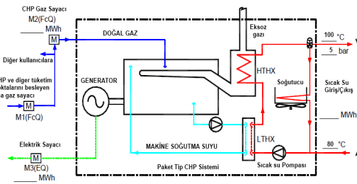
Şekil 1: Gaz Motorlu Paket Tip Kojenerasyon Ünitesi Prensi Şeması
