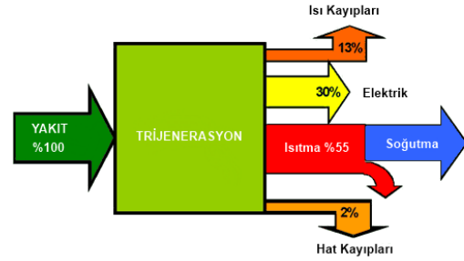
Şekil 4: Trijenerasyon Sistemi prensip gösterimi
