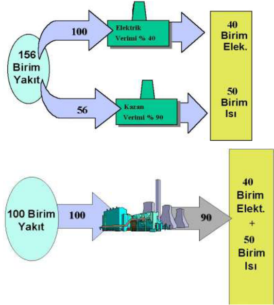
Şekil 2: Elektrik ve ısının ayrı ayrı ve birlikte üretilmesi halindeki yakıt giderleri
