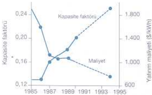
ŞEKİL 2: Rüzgar türbini kullanımı; şekilde kapasite faktörü olarak gösterilmiş; ortalama güç çıkışının rated (reyiç) güç çıkışına oranı ve Kaliforniya'daki rüzgar türbinleri için gerekli alt yapı yatırım maliyeti. U.S. Rüzgar gücü'nün (Windpower) dosyasına dayanarak, U.S. Rüzgar gücü'nün 33MW-S deyişken hızlı türbininin 1994 yılı maliyet ve kapasite faktörü tahmini. 1990'daki kapasite faktörü Kaliforniya'daki tüm rüzgar çiftlikleri için ortalamadır. Sadece Altamont Geçidi'ndeki artık eskimiş makinaların kullanıldığı rüzgar çiftliklerinin bulunduğu alan için bu değer 0.24, San Geronio Geçidi için kapasite faktörü 0.24 ve Tehachapi Geçidi için 0.19'dir.
