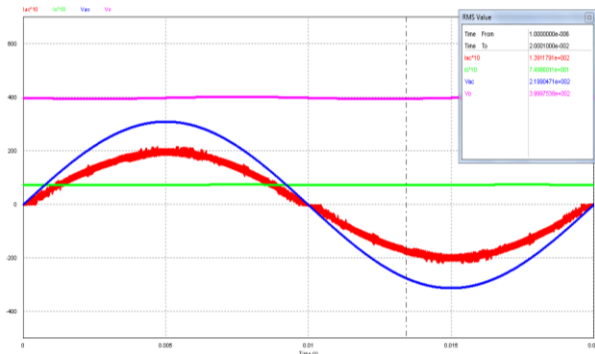
Şekil 10: Giriş ve çıkış akım-gerilim dalga şekilleri.
