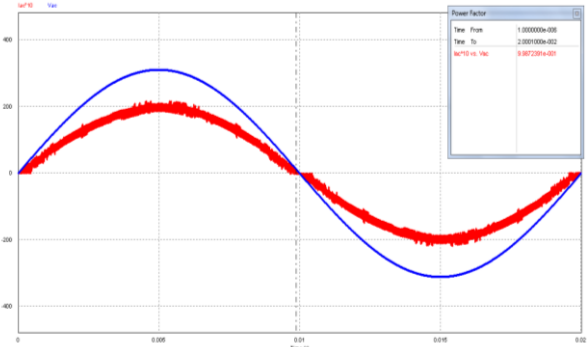
Şekil 11: Giriş akım ve gerilimine bağlı güç faktörü değeri.
