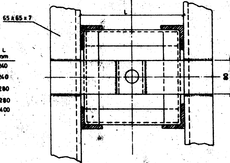
C - DETAYI ÖLÇEK 1/5 (KAFES DİREKLER İÇİN)
