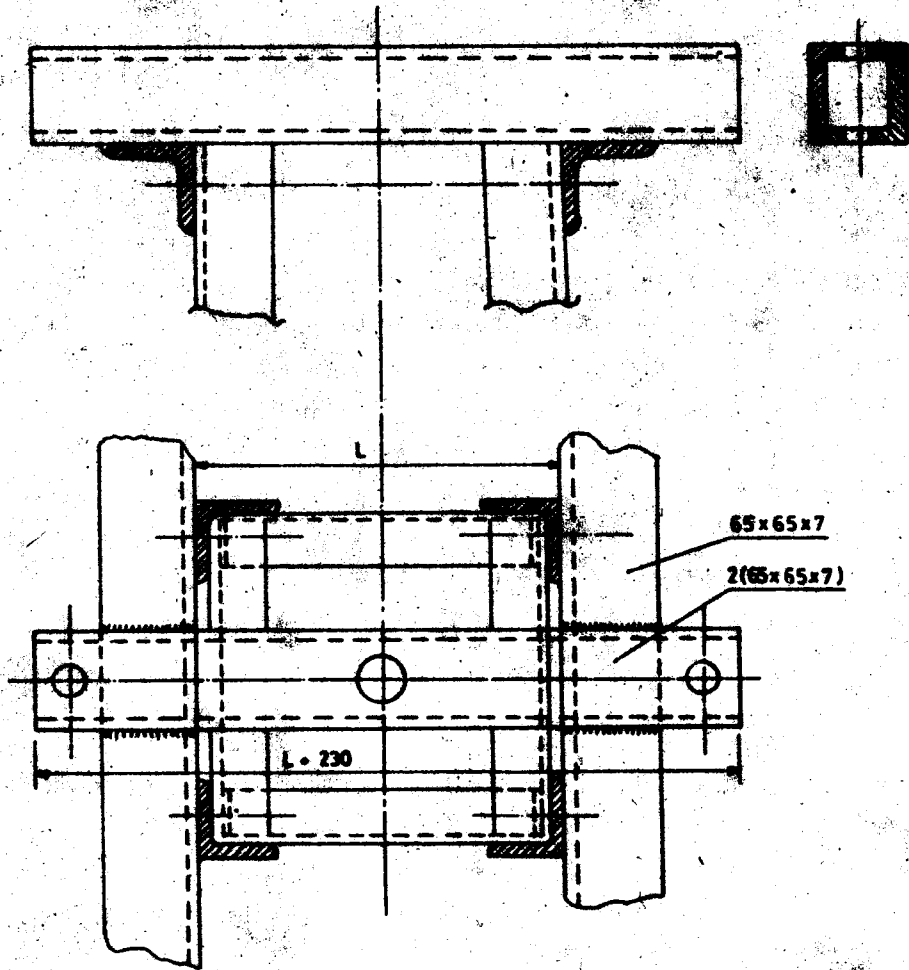
E - DETAYI ÖLÇEK: 1/5
