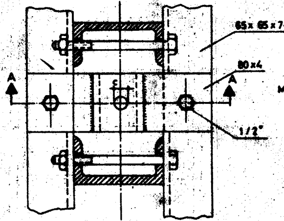
A - DETAYI ÖLÇEK: 1/5 (A DİREKLERİ İÇİN)
