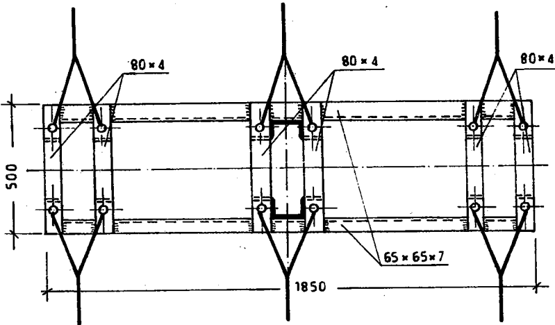
ÇİFT MESNET İZOLÂTÖRLÜ TRAVERS
