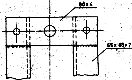
B - DETAYI ÖLÇEK: 1/5 (A DİREKLERİ İÇİN)
