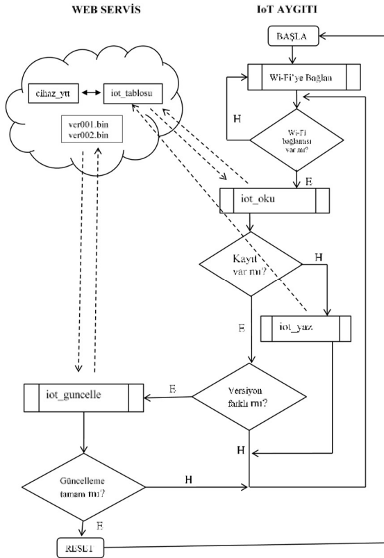
Şekil 6: Önerilen Uzaktan Yönetim Sisteminin Çalışma prensibi
