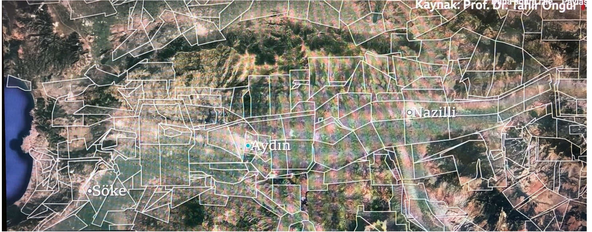
ŞEKİL -1 : BÜYÜK MENDERES GRABENİ - MTA RUHSAT SAHALARI
