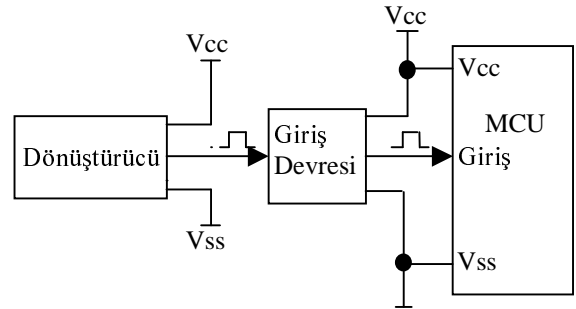
Şekil 1. Dönüştürücülerden Gelen İşaretin Giriş Devresi Aracılığıyla Mikrodenetleyiciye Aktarılmasının Blok Diyagramı
