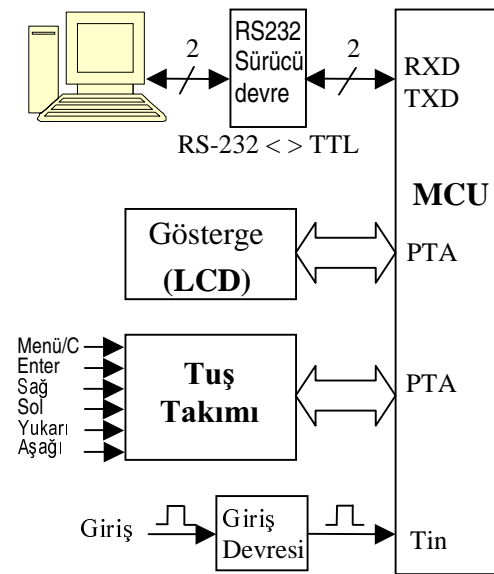
Şekil 6. Sistemin Blok Diyagramı
