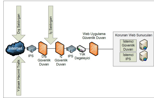
Şekil 3 Katmanlı Savunma için Mantıksal Yapı
