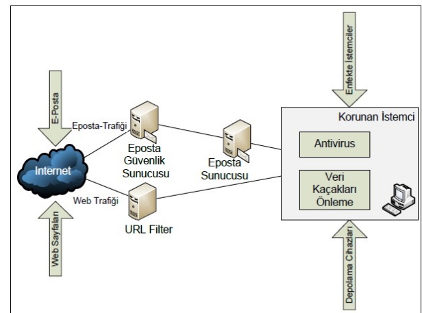
Şekil 4 Zararlı Yazılım Geliş Yolları ve Önlemler
