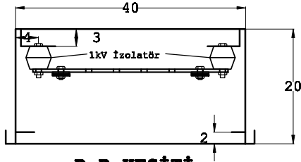
B-B KESİTİ
