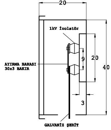
A-A KESİTİ
