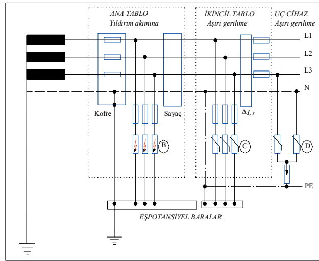
TN-C-S şebeke
