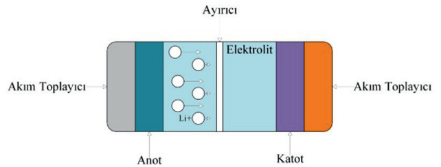
Şekil 1. LİB'lerin yapısı
