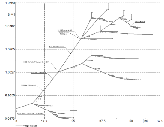
Şekil 7. Senaryo 4 sonucunda Kozluca Fideri Gerilim Profili
