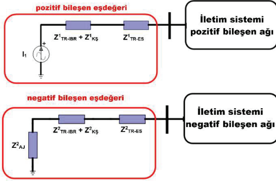
Şekil 9: DFIG tipi IBR'lerin (geleneksel CSC) pozitif ve negatif bileşen ağ eşdeğerleri.
