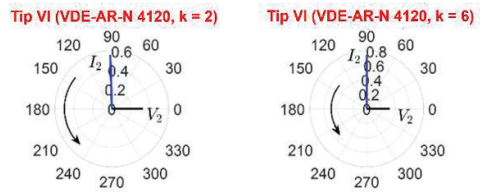
(b) SJ, Tip III ve Tip IV IBR'lerin V_2 ve I_2 fazörleri
