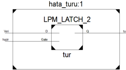
Şekil 3: Hata Modeli Belirleme Devresi.
