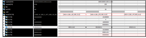
Şekil 10: r3 kaydedicisine gelen hatanın davranışsal simülasyonu
