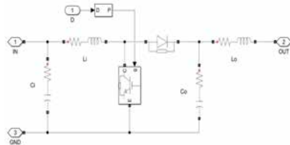
Şekil 5: Yükseltici dönüştürücü.
