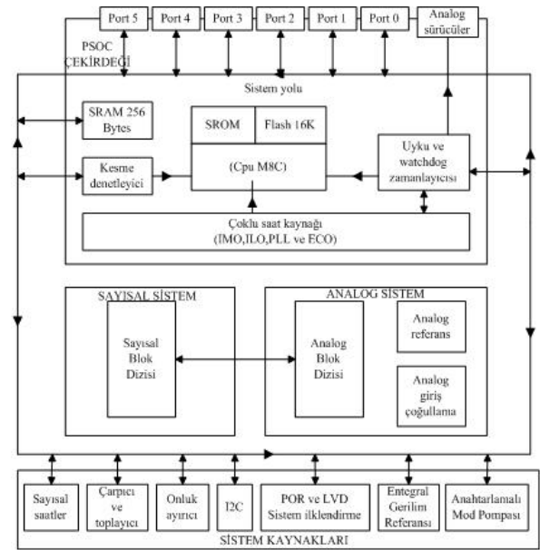
Şekil 4 Cypress 27443 Sistem Mimarisi
