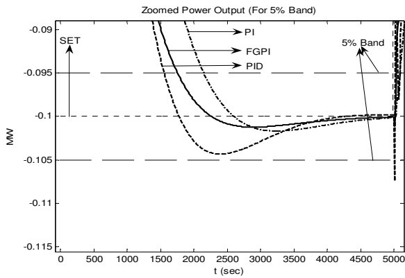
Şekil 4.2: Güç çıkışının %5'lik band için yakınlaştırılmış hali
