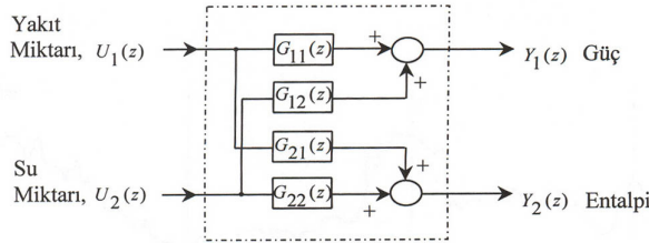
Şekil 2.3: Kullanılan santral modelinin blok diyagramı
