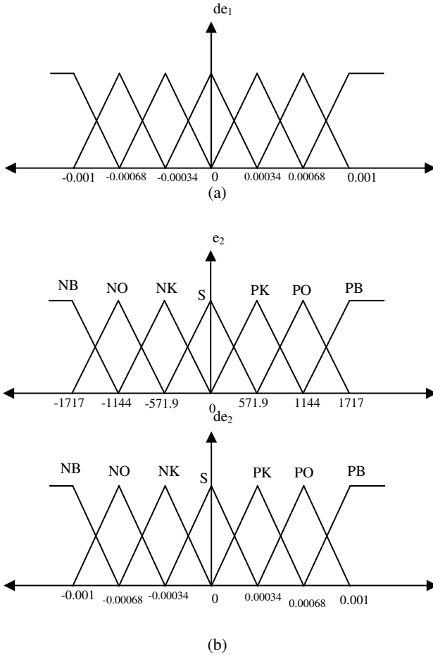
Şekil 3.2: Kullanılan giriş değişkenlerinin aralıkları (a) Güç çıkışı, (b) Entalpi çıkışı
