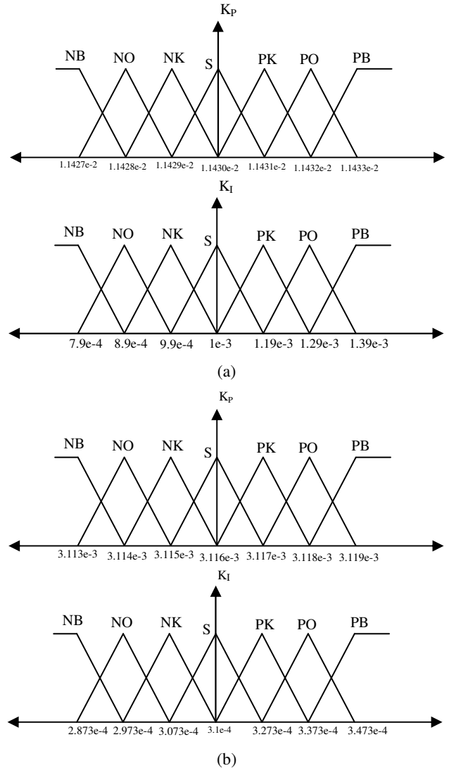
Şekil 3.3: Kullanılan çıkış değişkenlerinin aralıkları (a) Güç çıkışı, (b) Entalpi çıkışı
