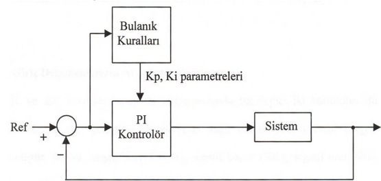
Şekil 3.1: Bulanık Kazanç Programlama Şeması
