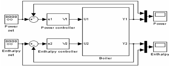
Şekil 4.1: Modeli alınan sistemin kontrol blok diyagramı
