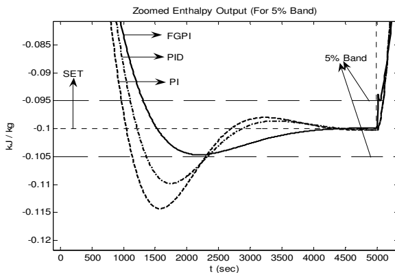
Şekil 4.3: Entalpi çıkışının %5'lik band için yakınlaştırılmış hali
