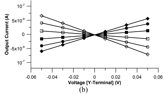
Fig. 4. DT MOS multiplier output current respect to input voltage. a) I_o-V_x , ( V_y parameter -50mV...+50mV ), b) I_o-V_y , ( V_x parameter -50mV...+50mV )
