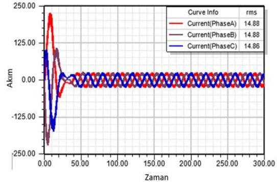
Şekil 10: Referans motor akım-zaman grafiği
