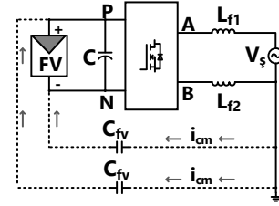
Şekil 5. Transformatörsüz FV eviricide kaçak akım akışı.
