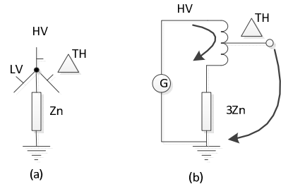
Fig. 6. YNd transformer configuration
