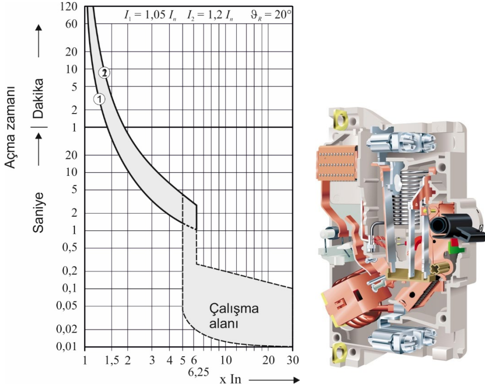
Şekil 10: Seçici kesicinin çalışma prensibi [Kaynak Hager]
