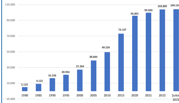
Türkiye Kurulu Gücünün Yıllar İtibarıyla Gelişimi (MW / 1980 - Şubat 2023)
