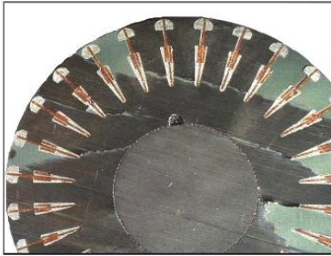
Şekil 5: Bakır çubuk üzerine alüminyum döküm yapılmış oluk yapısı [15]
