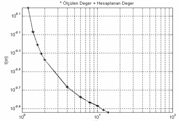
Şekil-4 Orta ters-zamanlı koruma eğrisi
