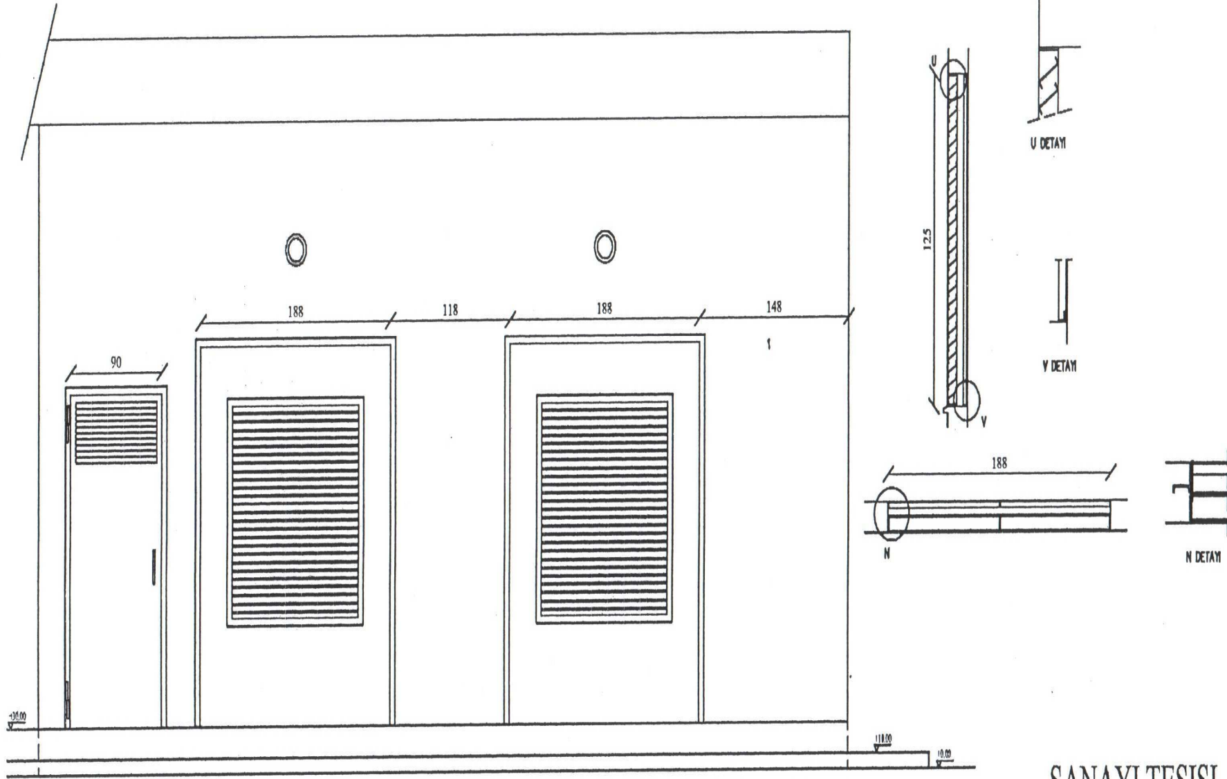
GENERATOR MERKEZİ KAPI-HAVALANDIRMA PANJURU DETAYI Ö:1/20
