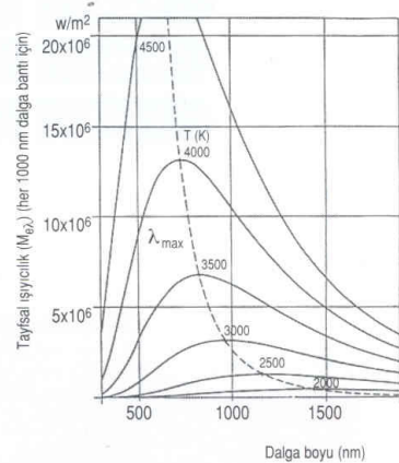
Şekil: 1- Kara cismin ışıma eğrileri
