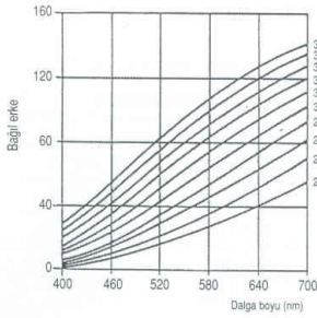
Şekil 2: Akkor lambanın değişik sıcaklıklardaki (K) ışınım tayfları
