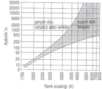
Şekil: 6- Aydınlik düzeyi - renk sıcaklığı ilişkisi
