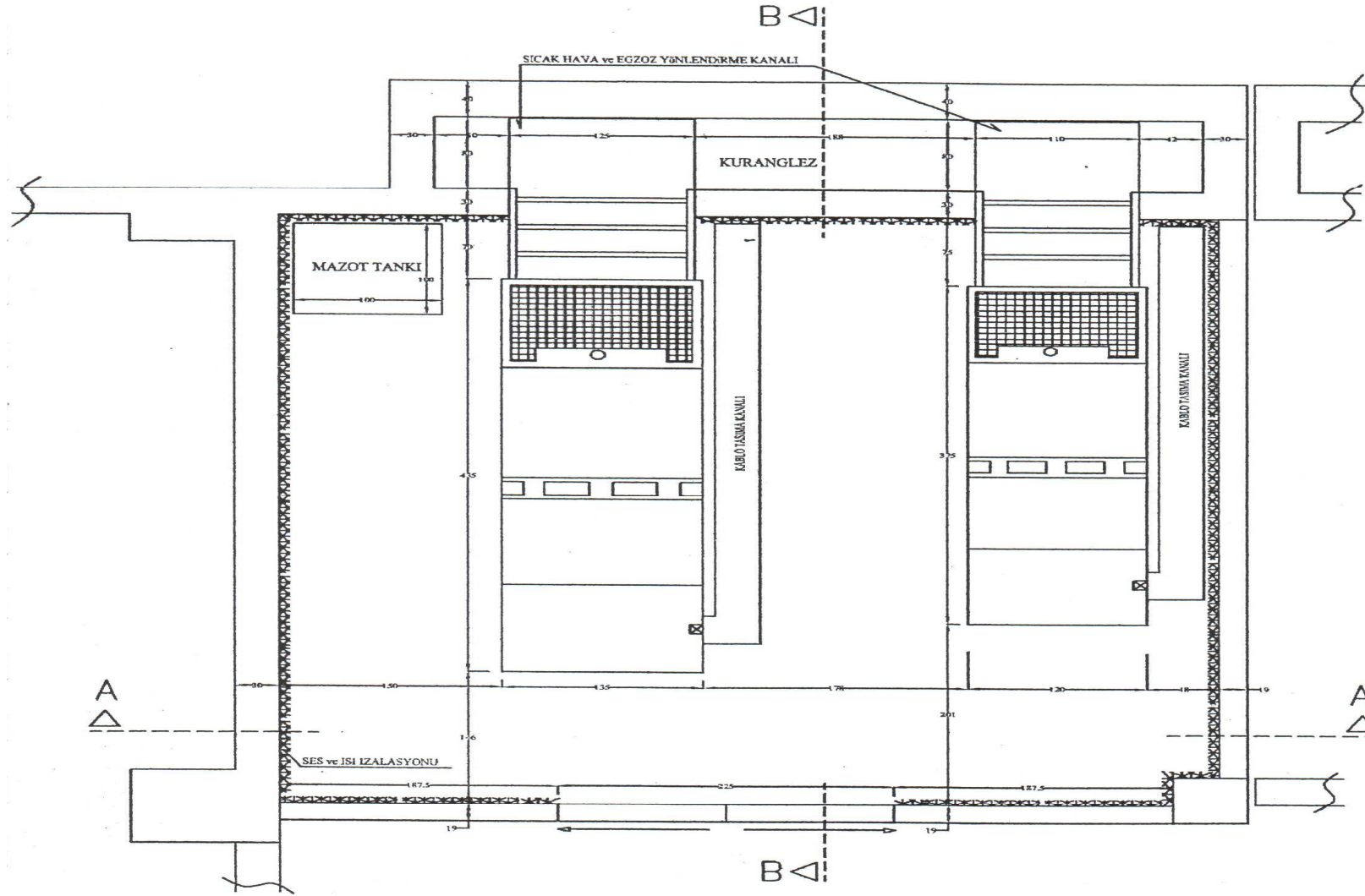
PLAN Ö:1/20 KAT ARASI
