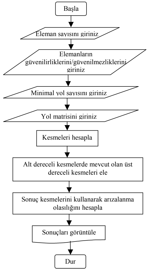
Şekil 1 Geliştirilen programın akış diyagramı[4]
