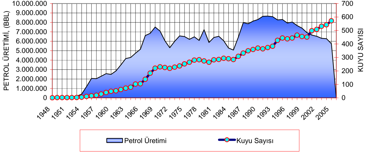
Şekil 2. Batman Bölgesi'nin Yıllara Göre Petrol Üretimi ve Kuyu Sayısı
